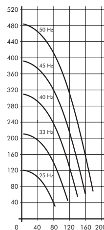
Disposición tándem mediante convertidor de frecuencia
